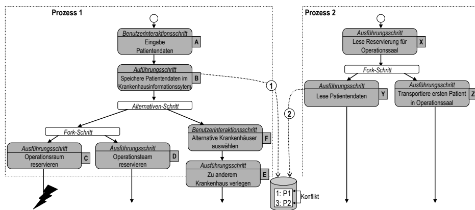
Abbildung 4: Beispiel für das Rücksetzen
