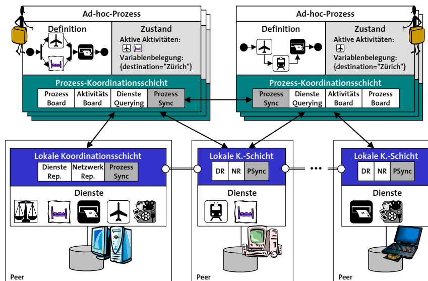
Abbildung 3: Aufbau des AMOR-Systems
