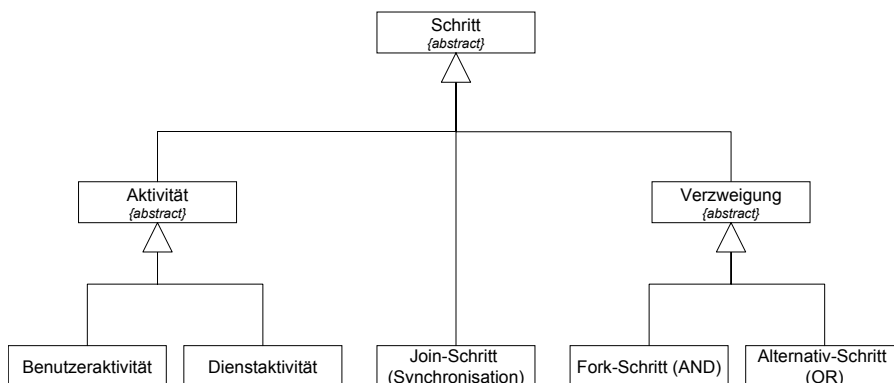
Abbildung 1: Arten von Prozessschritten
