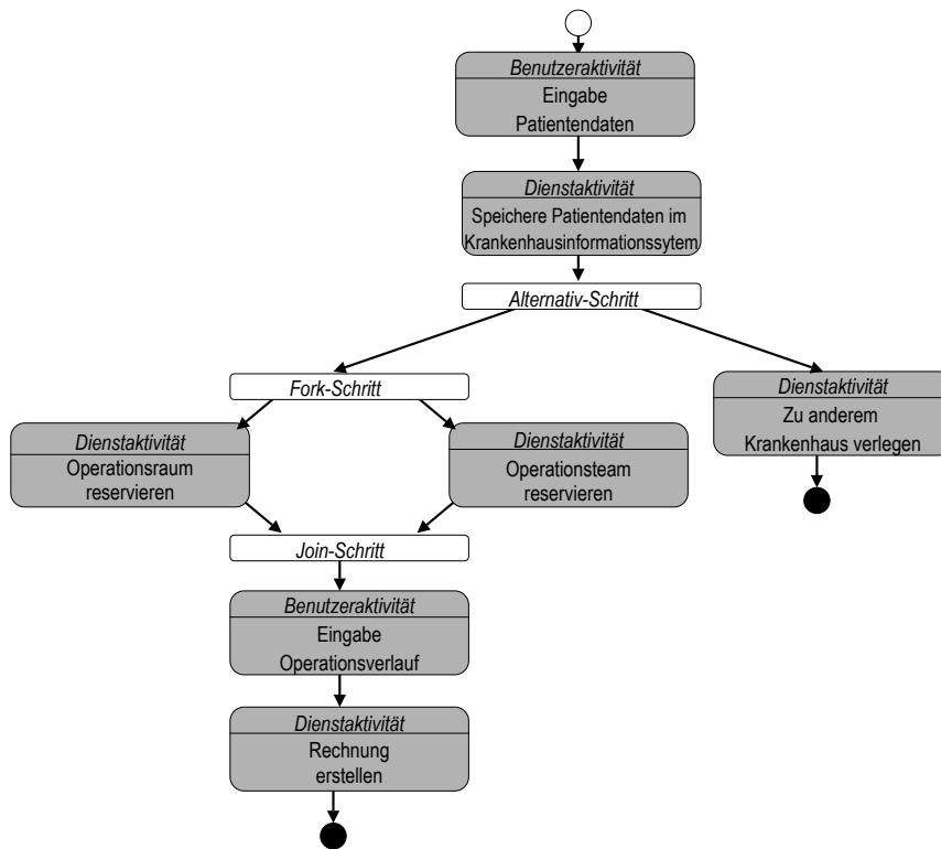
Abbildung 2: Spezifikation eines Ad-hoc-Prozesses
